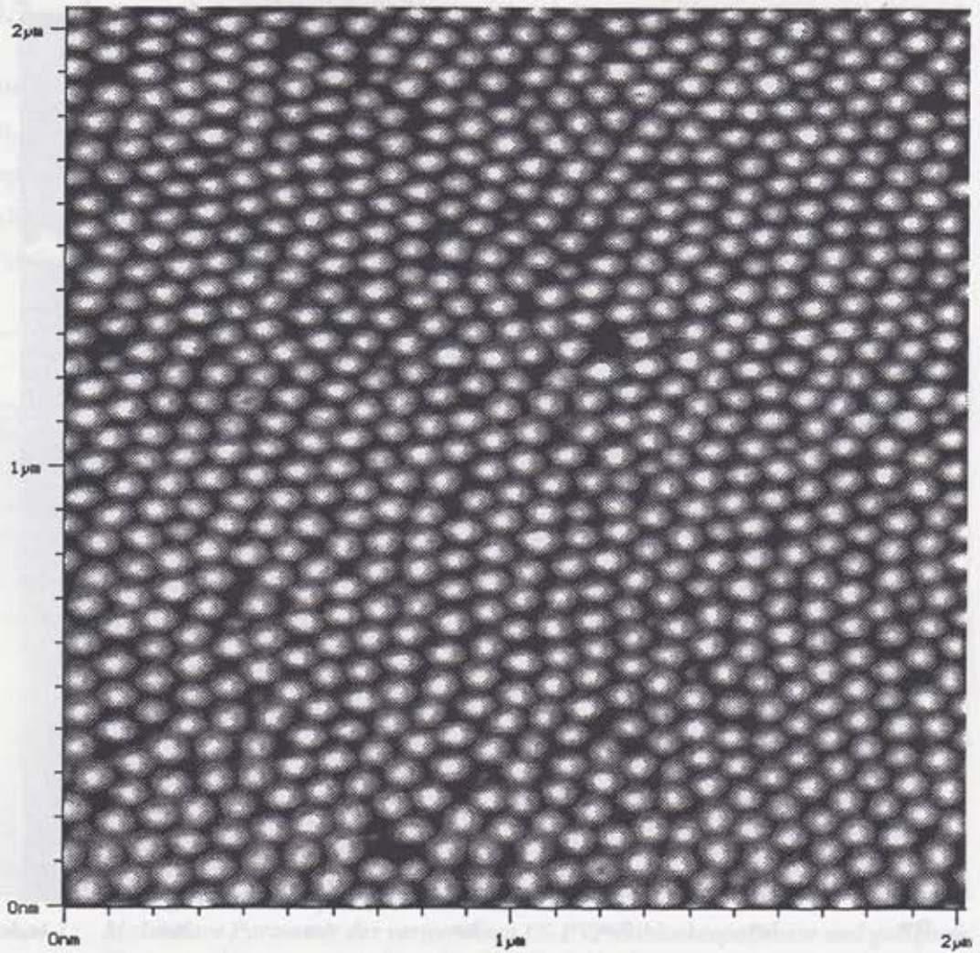
Abb. 4.5: AFM-Aufnahme eines 2 \times 2 \mu\text{m}^2 großen Ausschnitts einer aus Toluol adsorbierten PS-PVP-Diblockcopolymerschicht auf Glimmer; insbesondere sind hier die Korngrenzen und Punktdefekte zwischen den quasikristallinen Bereichen gut zu erkennen.
